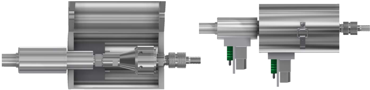
Abbildung 3: Montage der kleinen Heizung.
