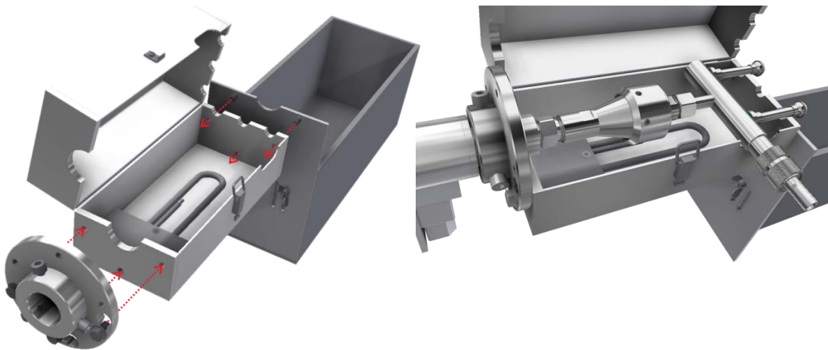
Abbildung 4: Montage der großen Heizung.
